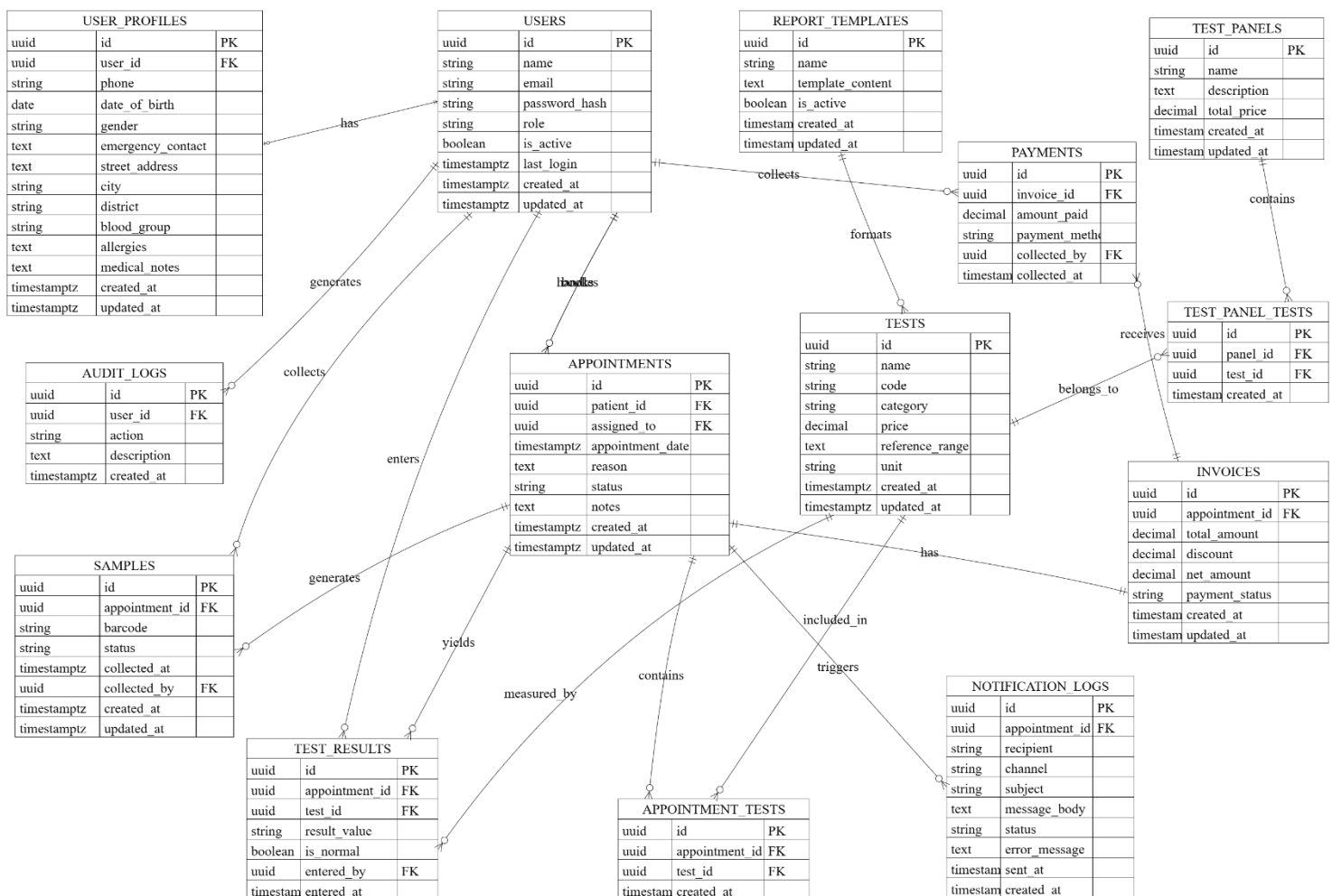
Figure 8: ER diagram
